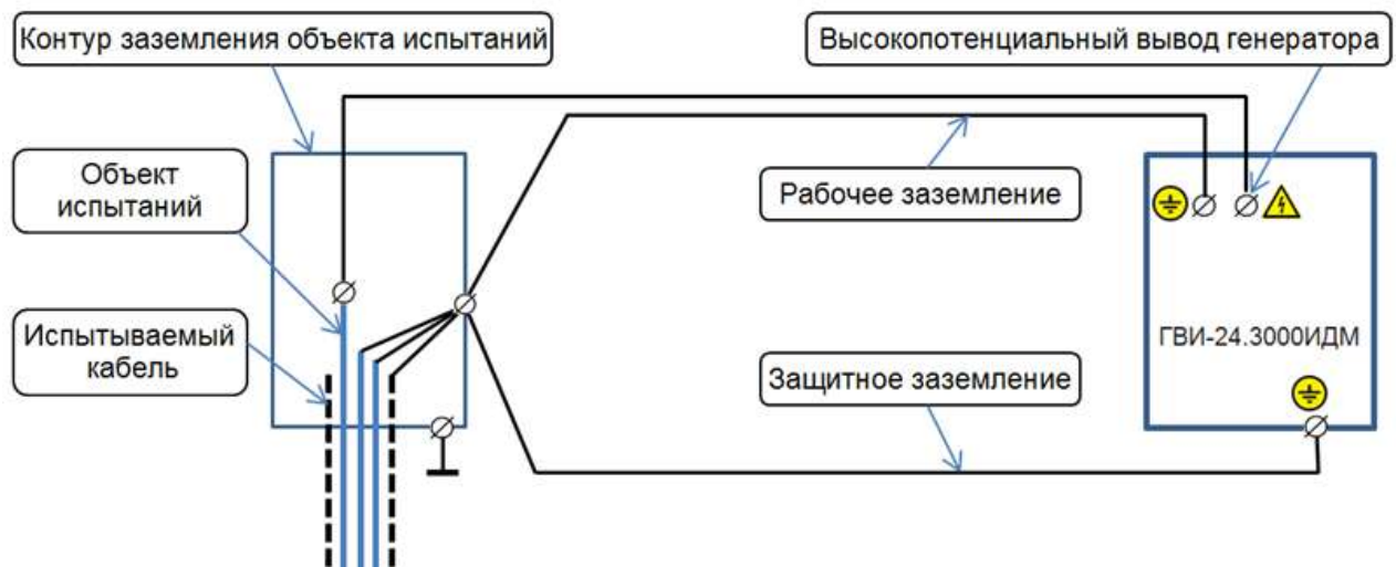
Схема 1 Подключение генератора к испытываемому кабелю.
